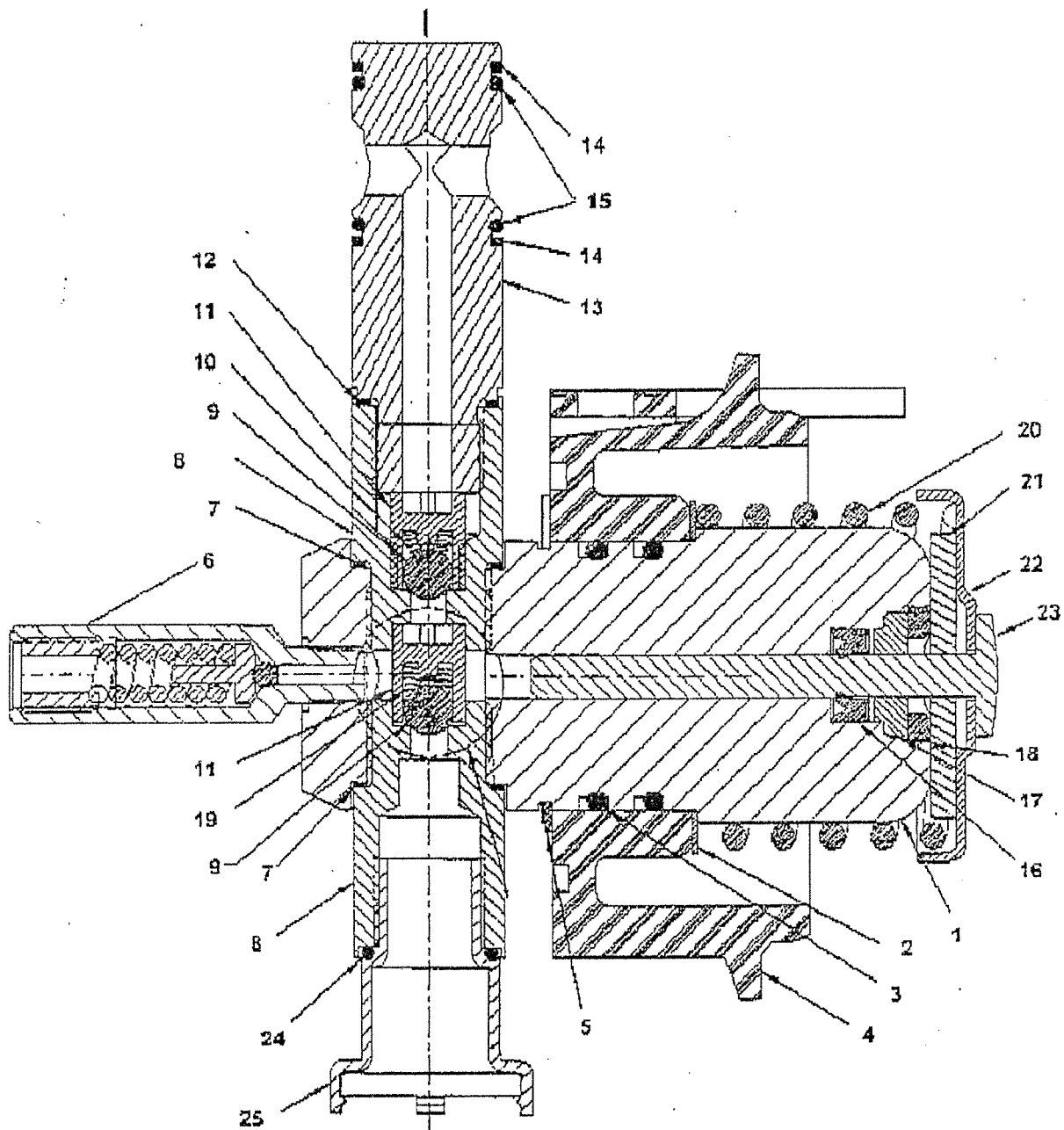
SECTION A-A
