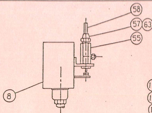
圧力開閉機詳細
