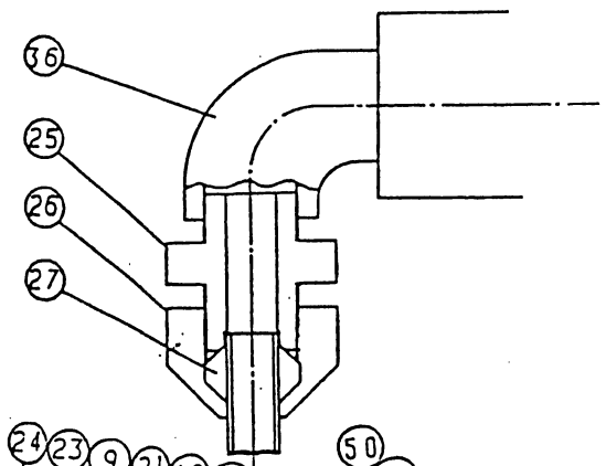
接続管接続部詳細
