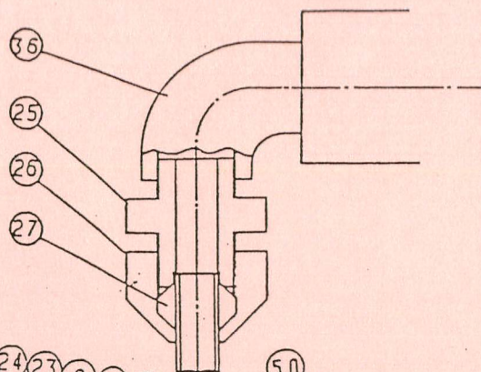
接続管接続部詳細
