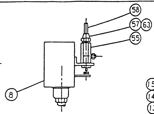
圧力開閉機詳細
