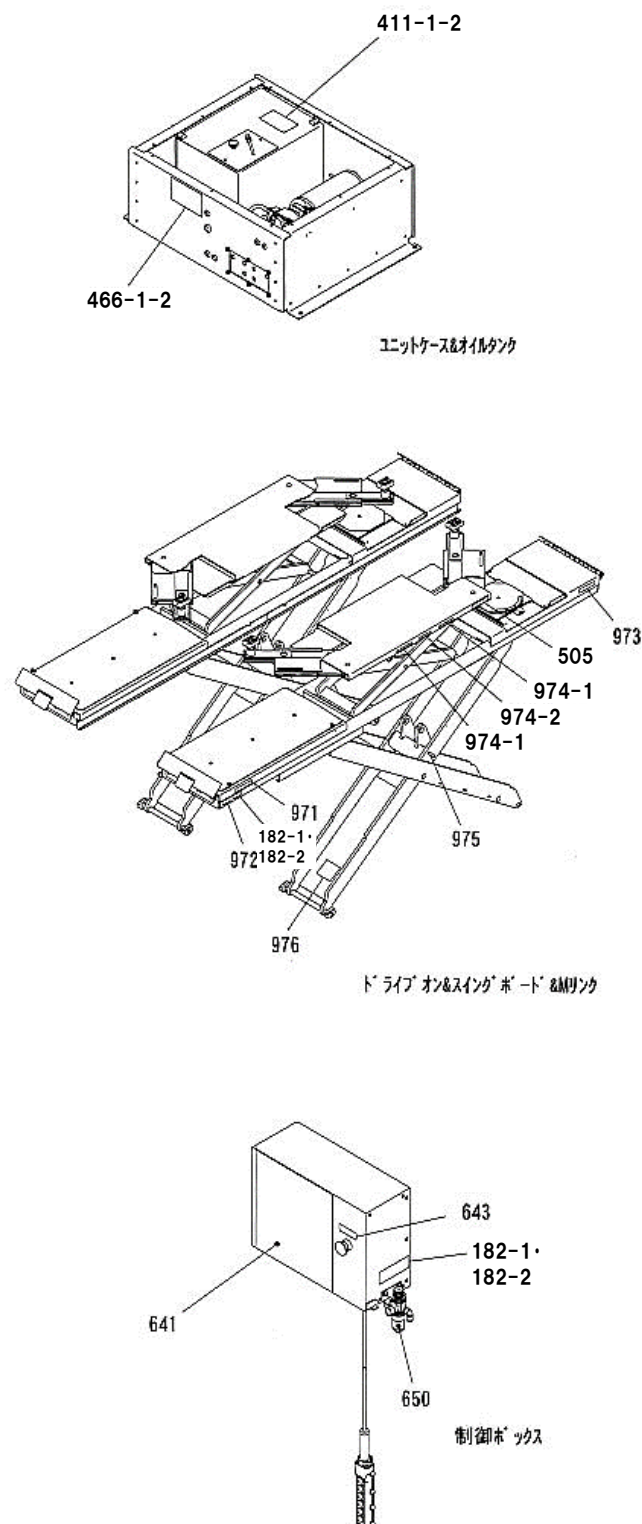
図番 411-1-2 11033511 エアハイカンシール (85mmX145mm)
