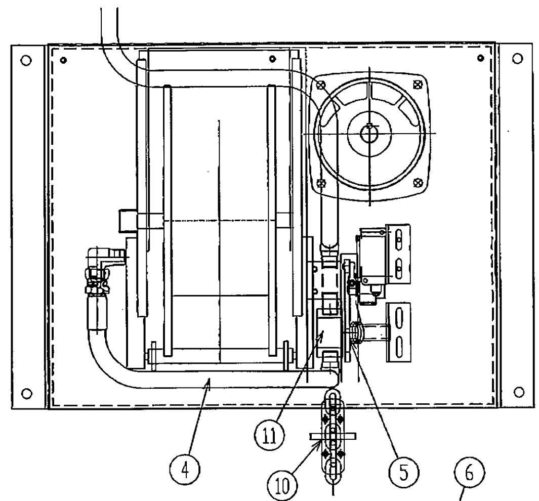
バルブブロックASSY
