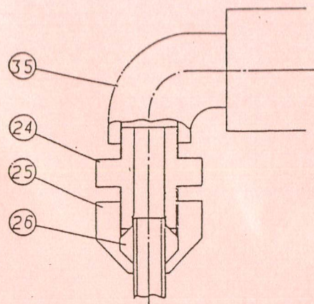
接続管接続部詳細
